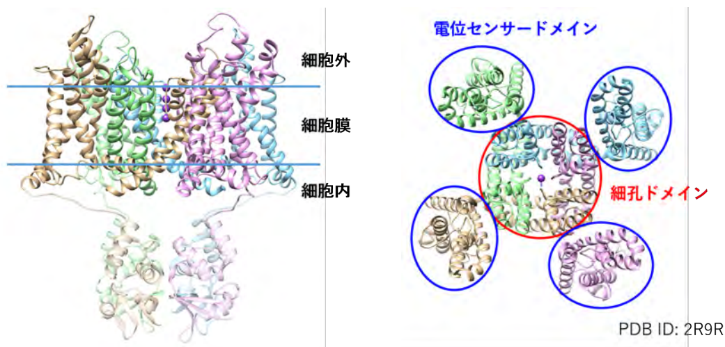
図4: カリウムイオンチャネルの立体構造
