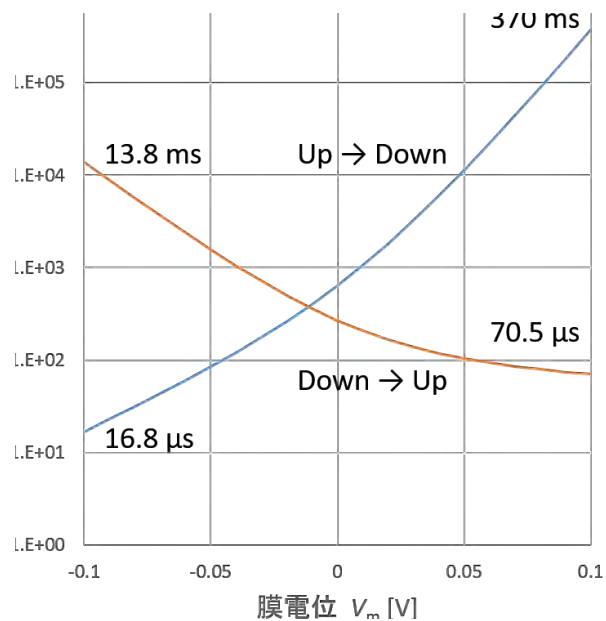
図7: Down状態・Up状態間の遷移に要する時間の膜電位依存性
